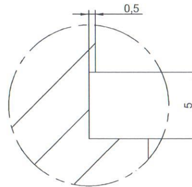
Szczegół A
