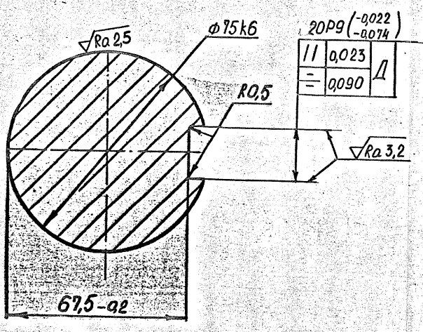
И-И (1:1) лист 1
