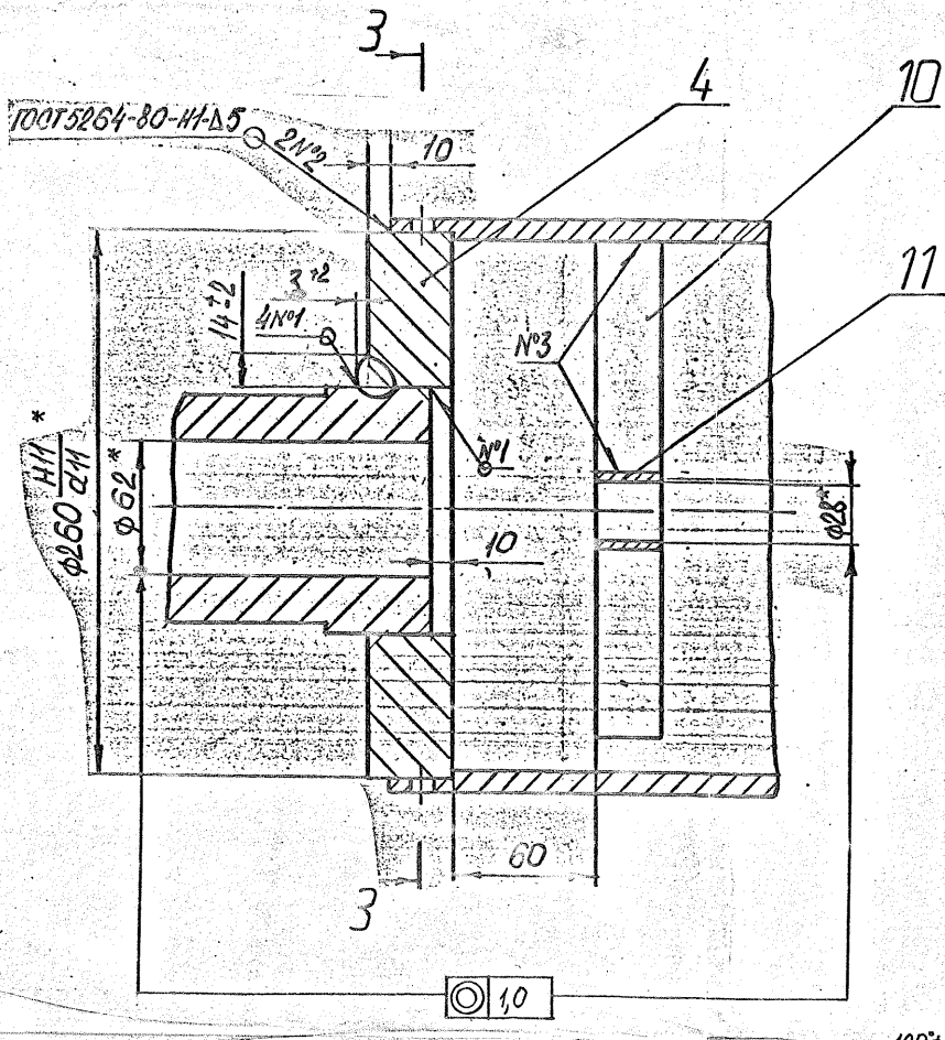
Г (1:2) лист 1
