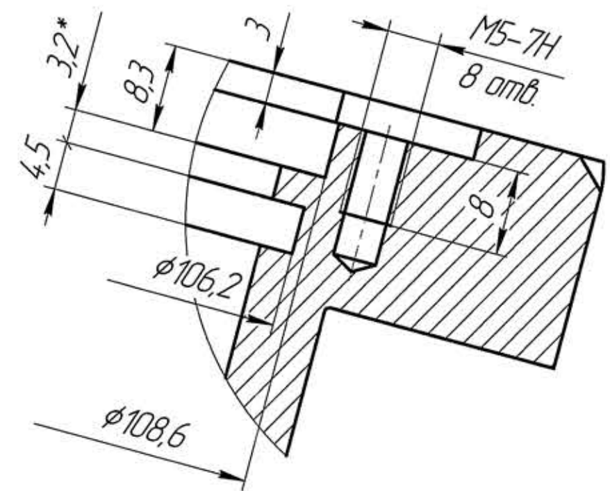
Г-Г (2:1)
