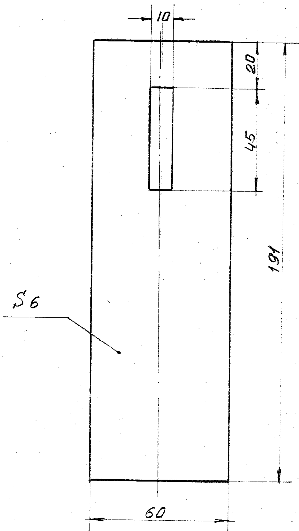
Ухо S6 Ст 20Х20Н14С2 Подвеска потолочн. труб котла №3
