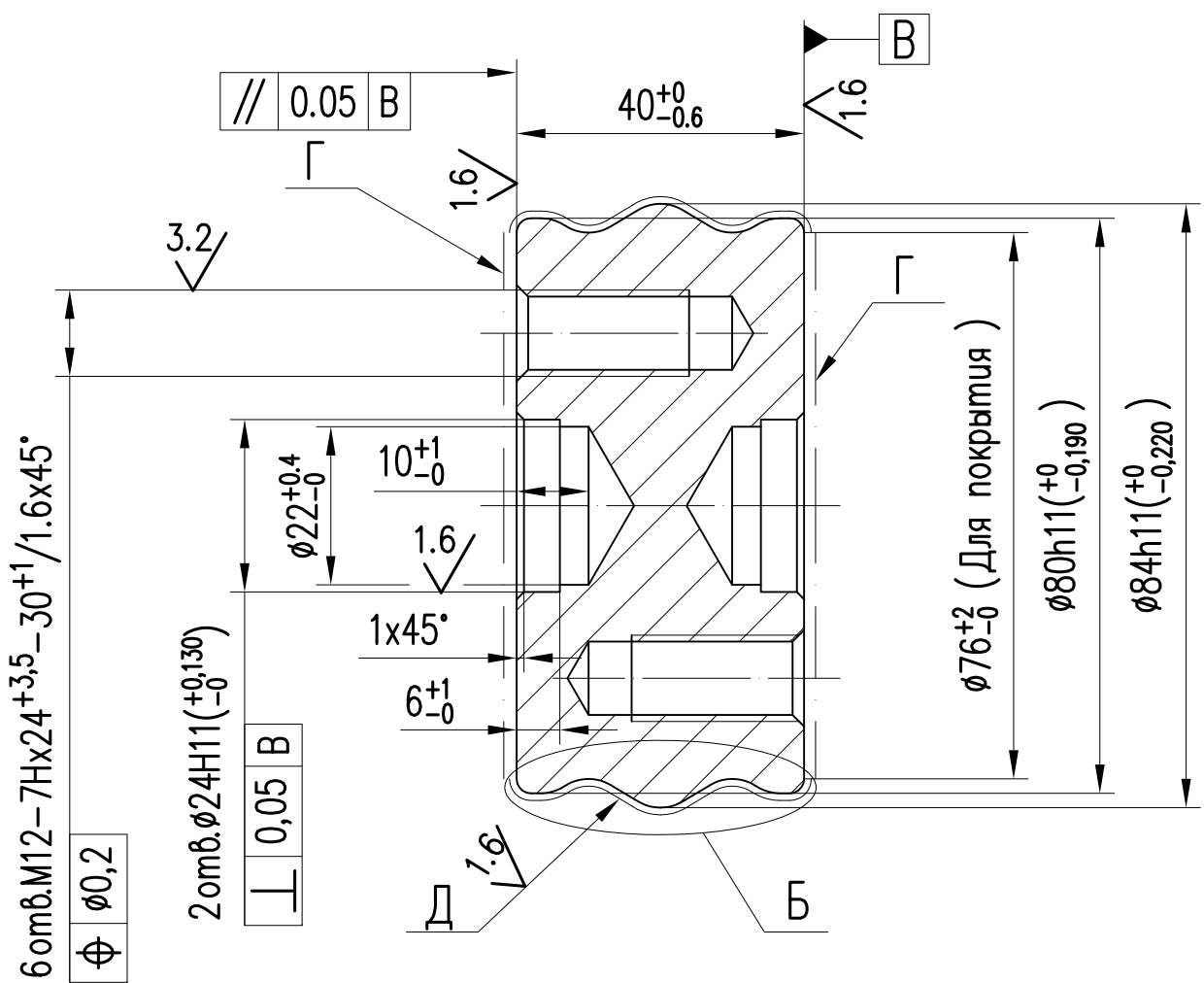
Рис.2 Остальное см. рис.1 A-A
