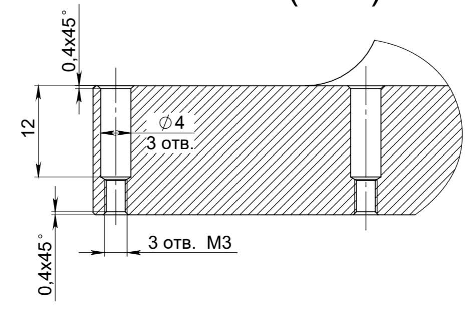
Е-Е (2 : 1)
