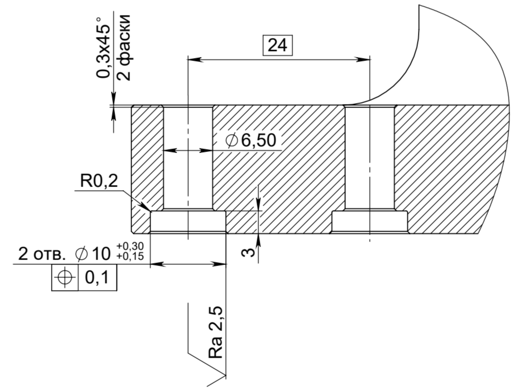
Е-Е (2 : 1)
