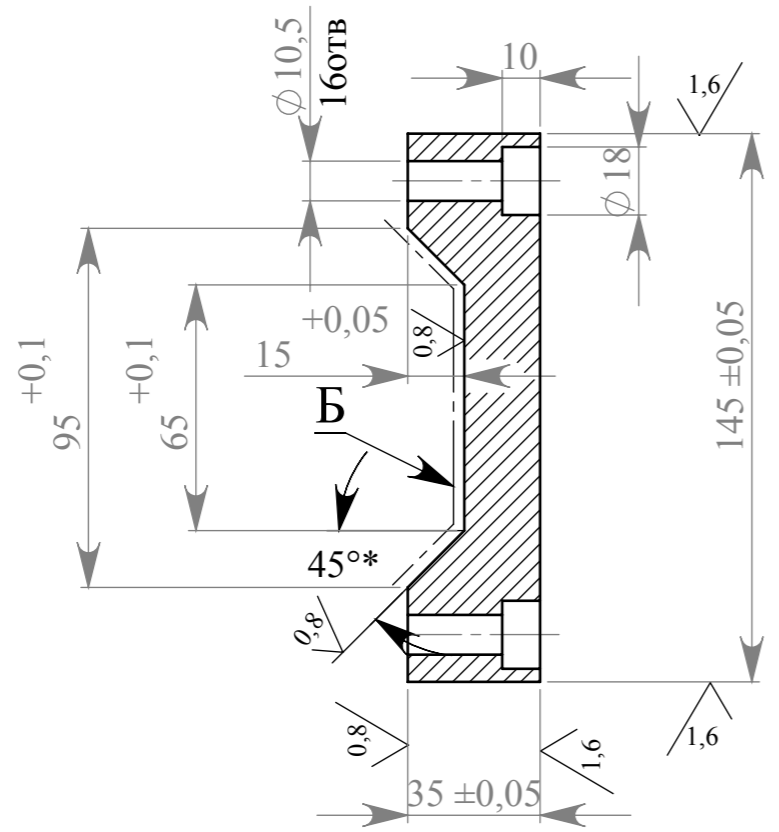
A-A (1 : 2)
