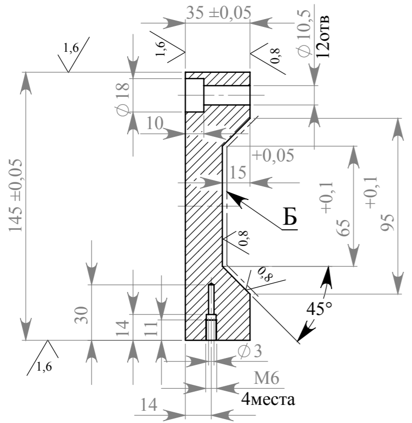
A-A (1 : 2)
