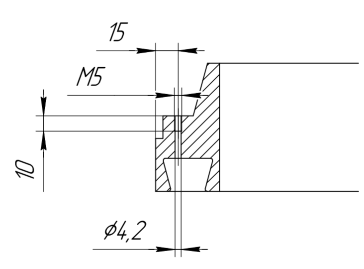
B-B(1:2,5) \odot
