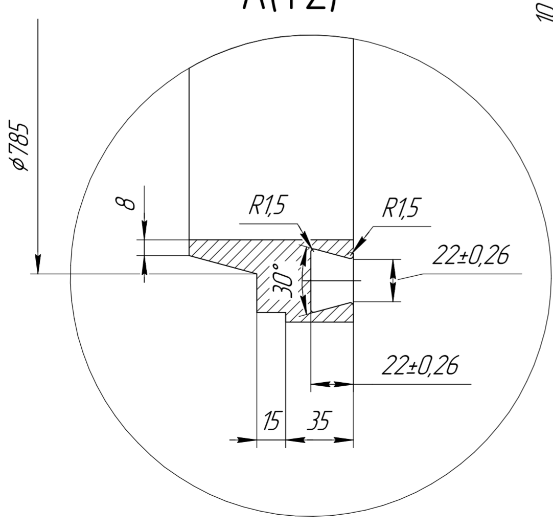
A(1:2)
