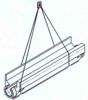
Схема строповки
