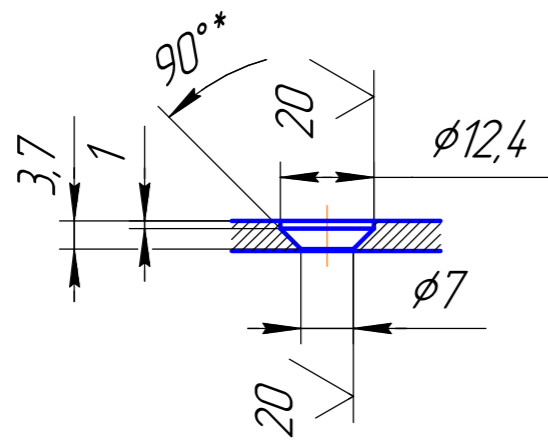
A-A(1:1) (12 мест)
