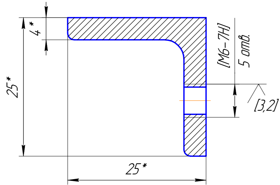
A-A(2,5:1)
