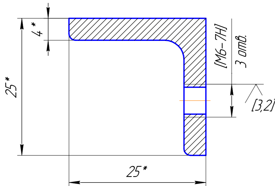
A-A(2,5:1)
