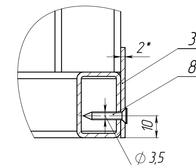
A-A (1:1)
