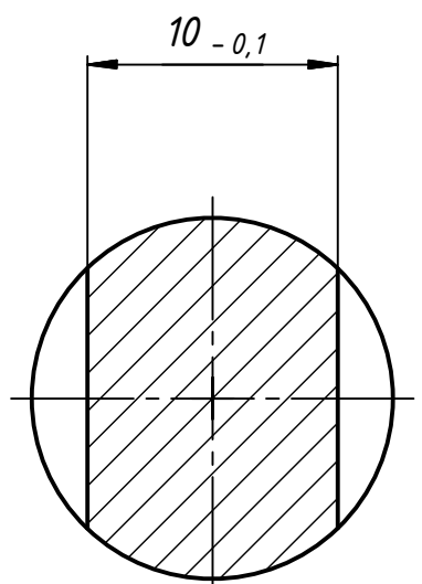
A-A (3:1)
