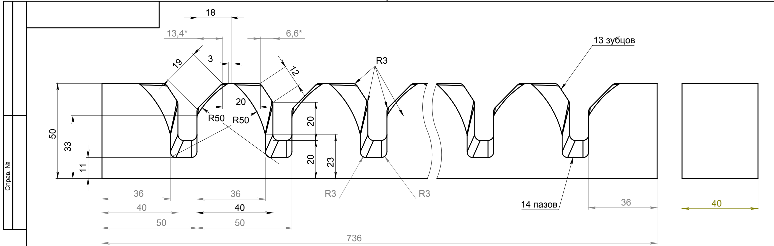
200124-09-Л - зеркальное отражение Остальное - см. 200124-09-П M1:5
