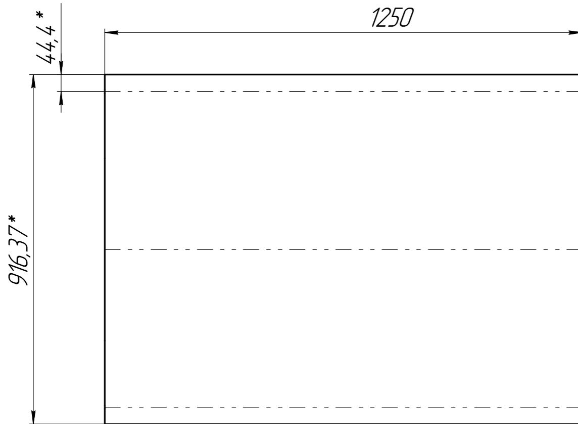
Развертка \Omega_2 (1:10)
