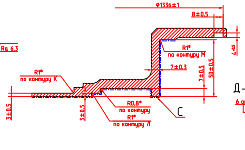
Б-Б (1:1) (3B,1B)
