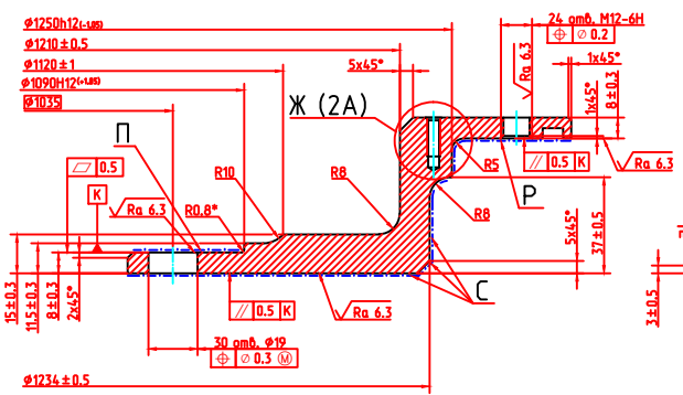
A-A (1:1) (3B)
