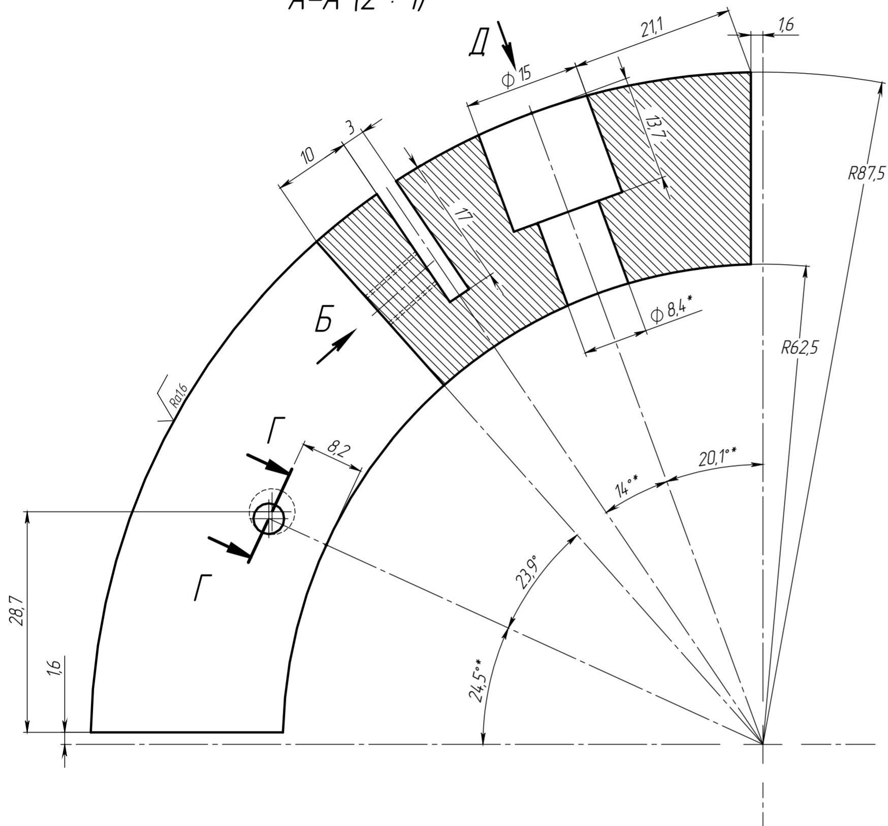
A-A (2 : 1)
