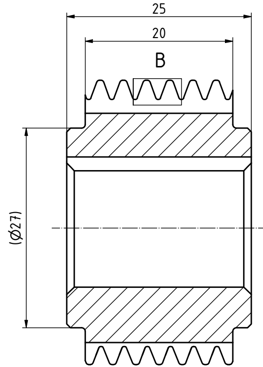
A-A ( 2 : 1 )
