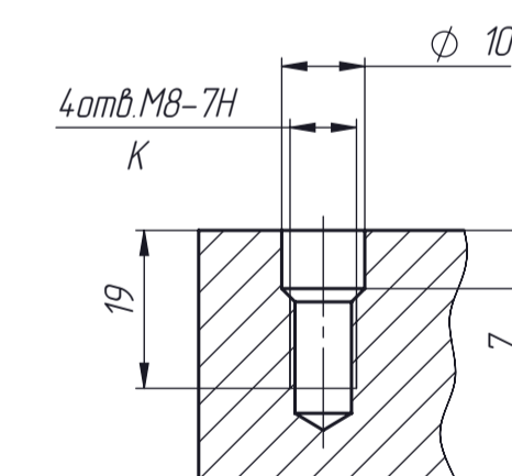
В-В(1:1)
