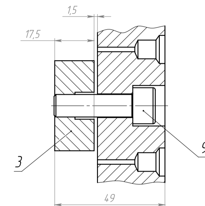
Б-Б(1:1) 8 элементов
