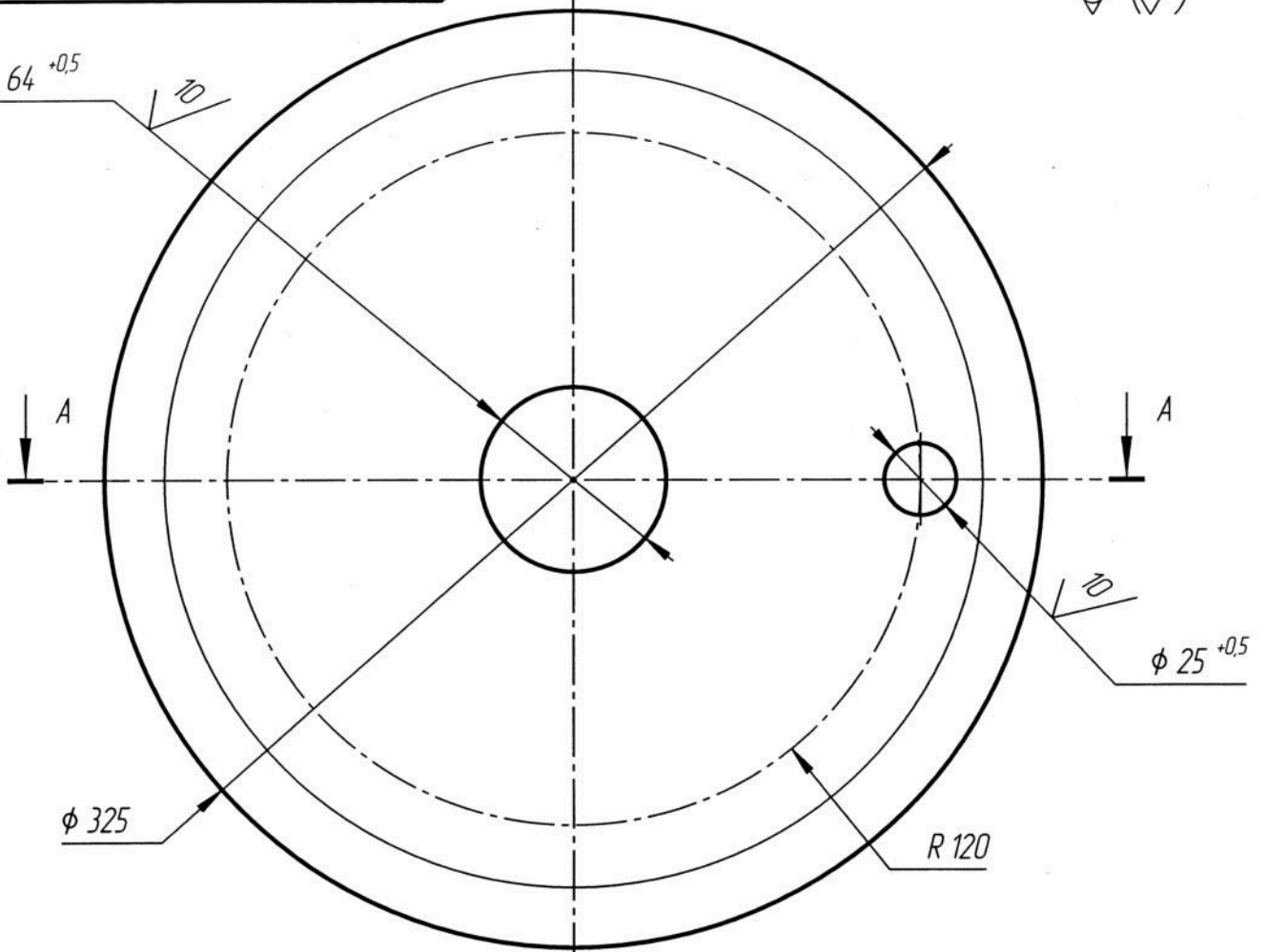
Вид сечения А-А Масштаб: 2:5
