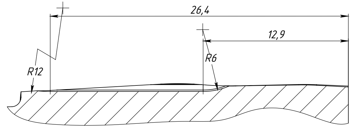
Б-Б (5 : 1)
