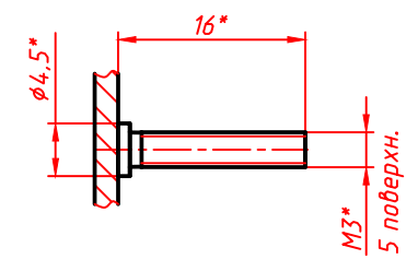
Б-Б (2:1)
