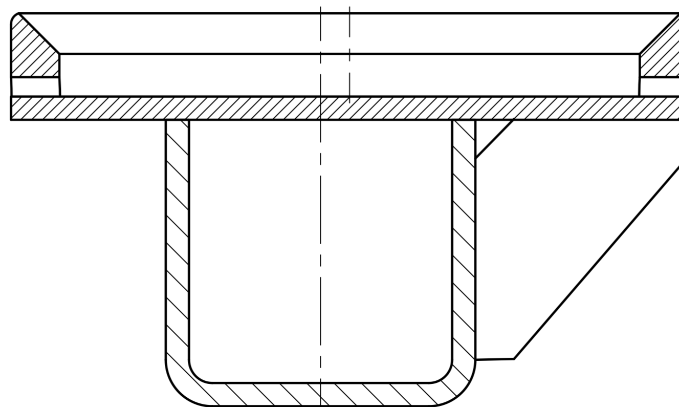
Б - Б (1:2)
