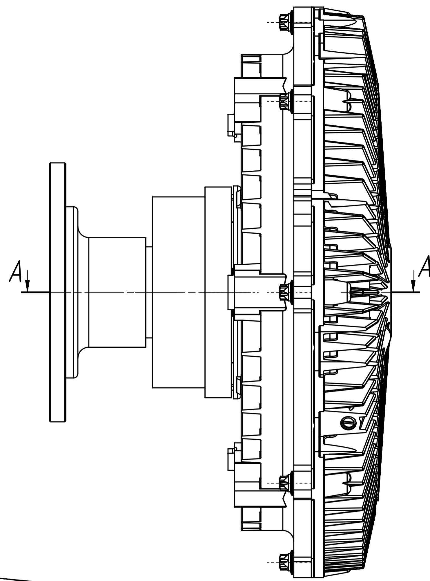
B (1:1) APBЦ.711318.001-Крышка поз. 6 не показана
