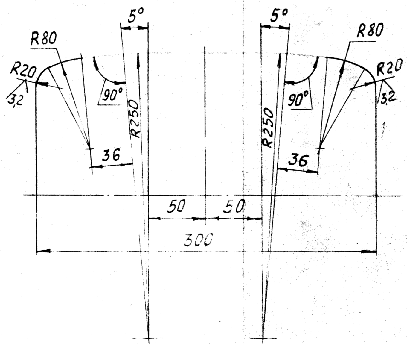
Построение профиля бочки валка
