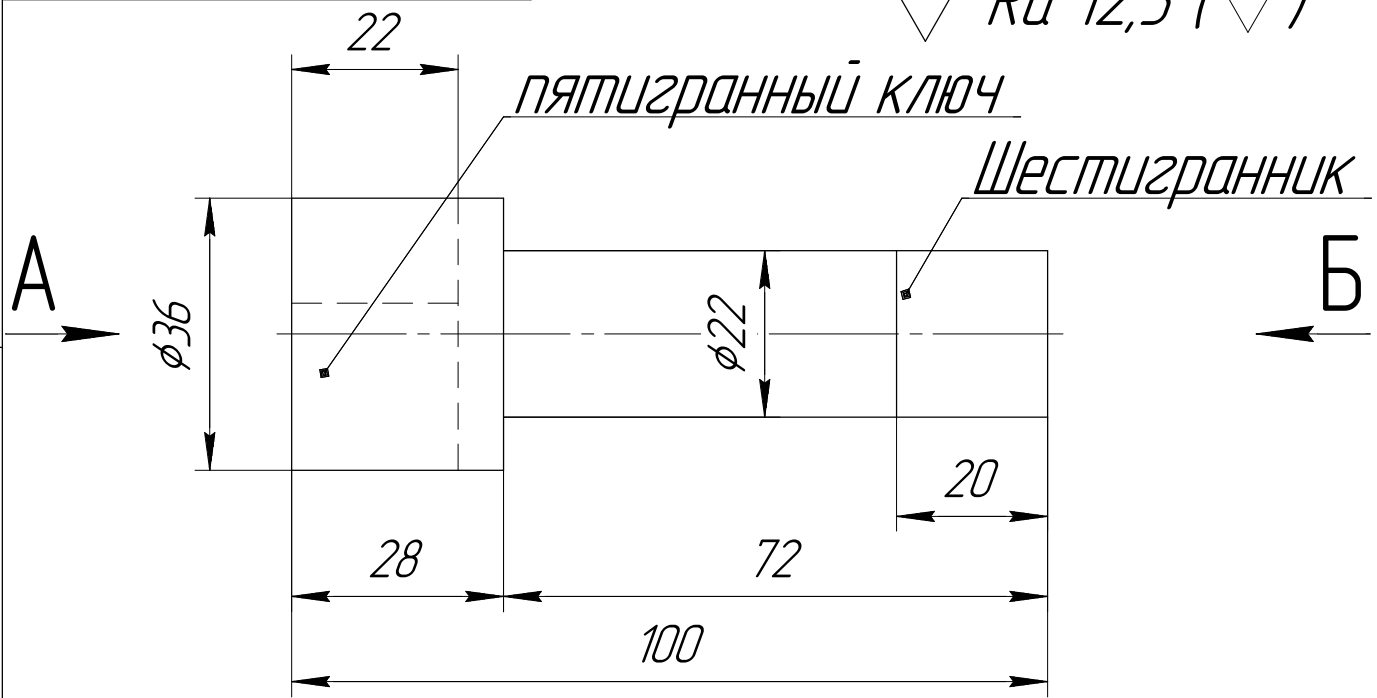
Вид А 5-гранная головка
