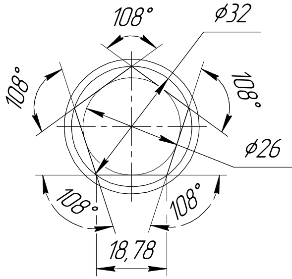
Вид А 5-гранная головка
