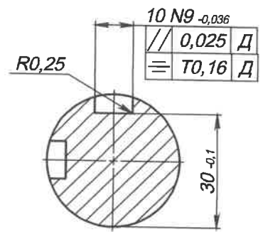
A-A (1:1)
