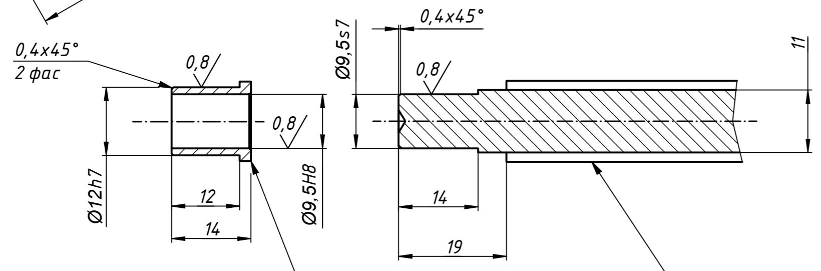
D-D (1.5:1)
