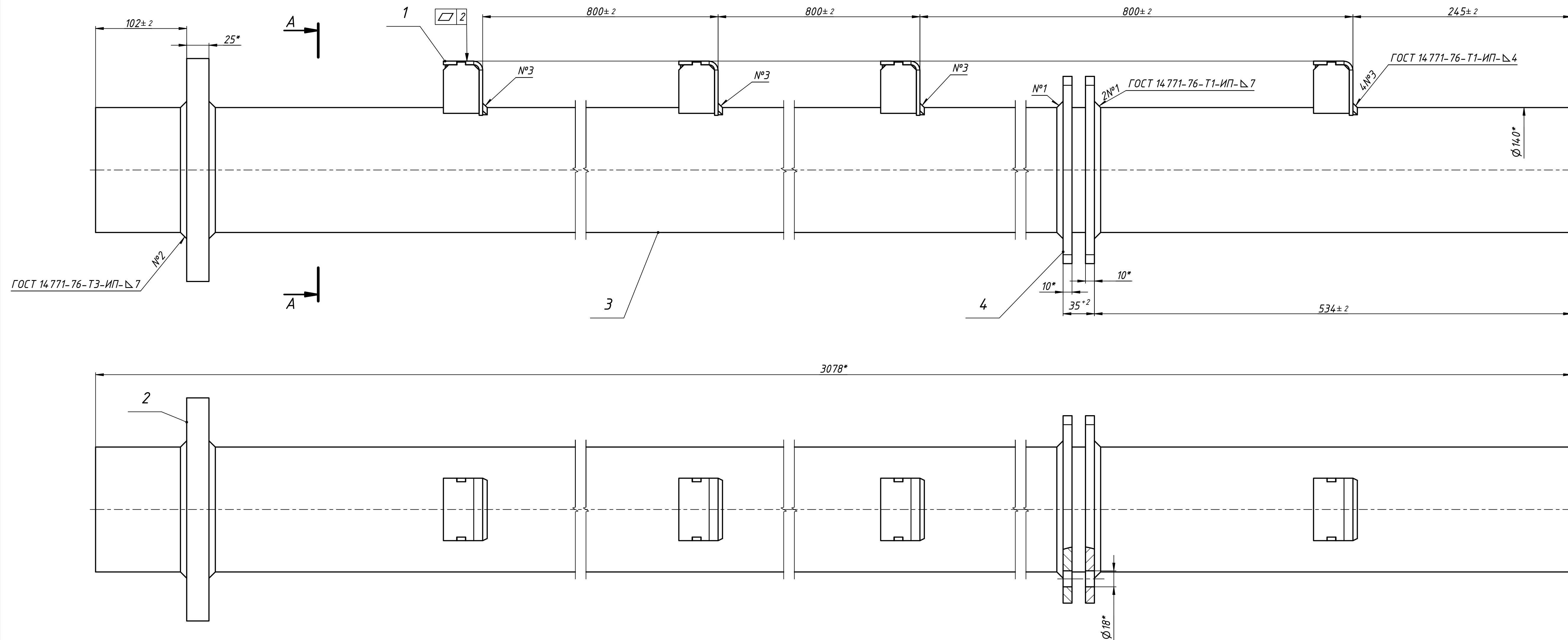
Рис.1 Корпус. Сварка
