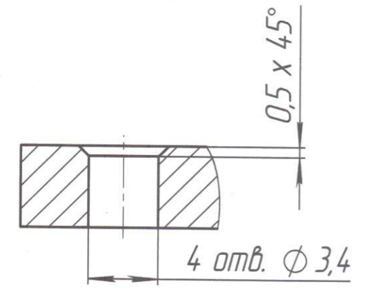
B-B (4:1)
