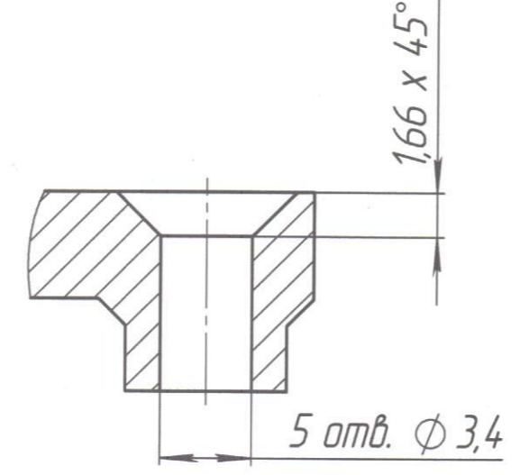
B-B (4:1)
