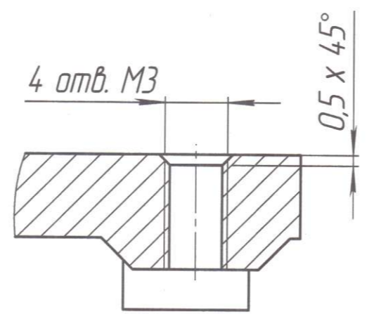
A-A (4:1)
